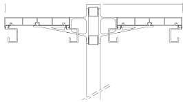
35X48 mit Mantelhaken | with coat hooks
