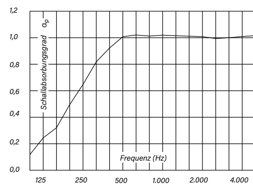
Schallabsorptionsgrad - Oktav-Mittenfrequenz
